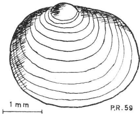
Abb. 18. Cyclestherioides franconica n. sp. (Holotyp, Slg Wzbg O 19 I 1 ).
